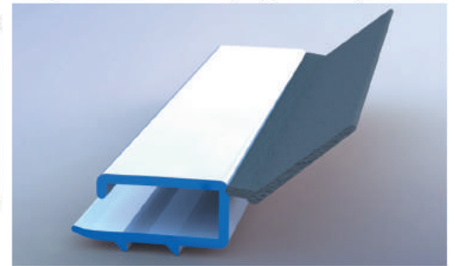
PB-SS profil uszczelki bramy segmentowej - szeroki
